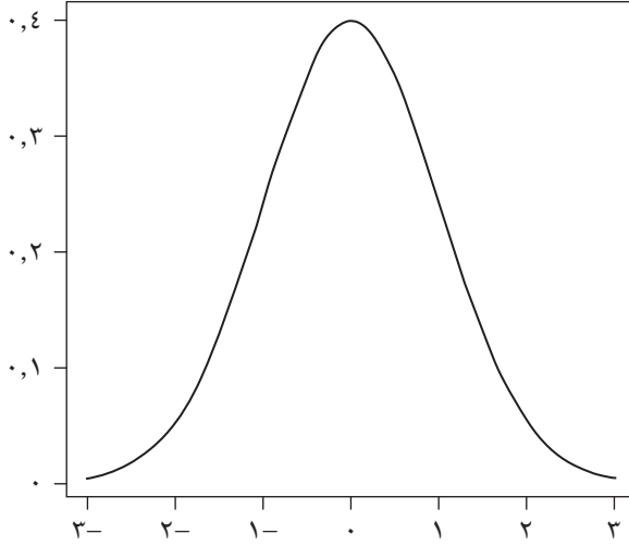
شكل ٤-٣: التوزيع الطبيعي.
